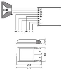
Technische Daten Osram PTi 35/220-240 I
